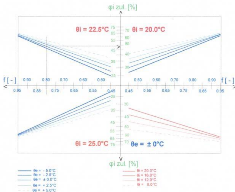
Bild 2: Zul. Raumlufffeuchte ( \phi_{i \text{ zul.}} ) je nach Temperaturfaktor ( f ) und Klima Zu Tabelle 1: Ablesung für d = 120 \text{ mm} : f_1 \sim 0.793 \rightarrow \phi_{i \text{ zul.}} \sim 48.3\%
