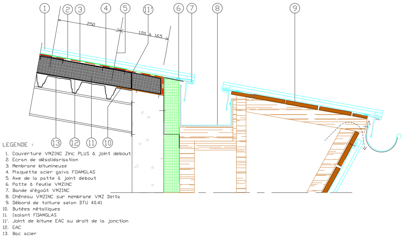
Figure 20 – Égout – Débord
